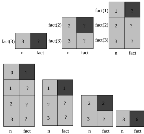
FIGURE 1 – La pile d'exécution
